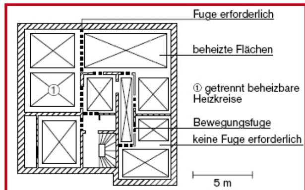
Abb. 4 Beispiel einer Flächenaufteilung durch Feldfugen
