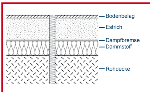
Abb. 1 Bauwerksfuge
