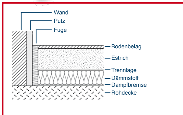
Abb. 3 Randfuge
