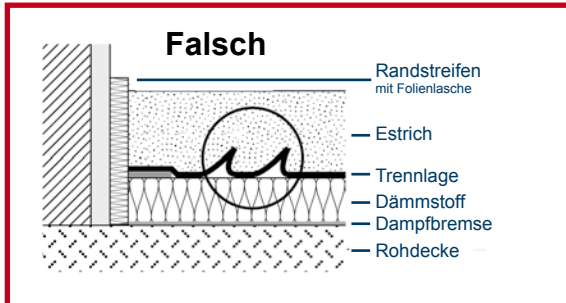
Abb. 5.3: Faltenbildung der Trennschicht: Mögliche Rissbildung im Fließestrich
