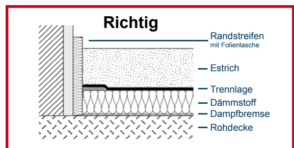
Abb. 5.2: Saubere Randausbildung, gleichmäßige Estrichdicke, glatt ausgelegte Trennschicht.
