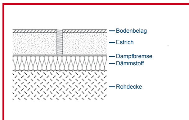
Abb. 2 Bewegungsfuge
