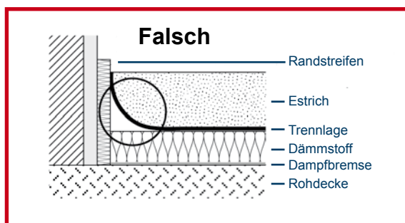
Abb. 5.1: Trennschicht als Hohlkehle ausgebildet: Gefahr des Ausbrechens bei Belastung, da Schwächung des Estrichs im Randbereich.
