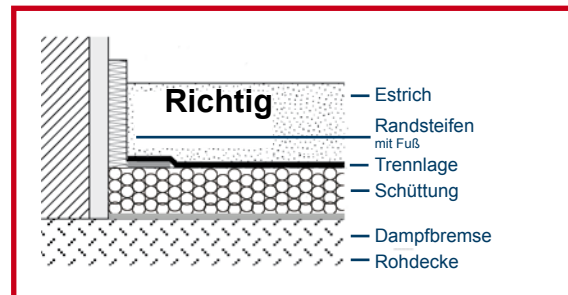
Abb. 5.4: Saubere Randausbildung durch Randstreifen mit Fuß, der direkt auf der Schüttung steht
